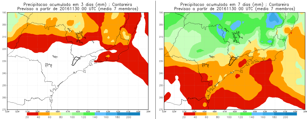
Figura 5. Previsão de precipitação acumulada em mm nos próximos 3 e 7 dias para a bacia de captação do Sistema Cantareira, segundo a previsão por conjuntos (média de 7 previsões semelhantes em que a cada previsão é iniciada com o estado da atmosfera ligeiramente diferente) do modelo numérico ETA/CPTec/INPE. A área da bacia de captação do Sistema Cantareira é indicada na Figura com linha preta espessa.
