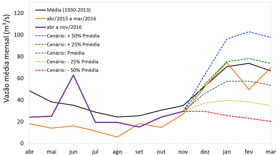
Figura 8. As linhas tracejadas apresentam cinco projeções de vazão média mensal afluyente, em m^3/s , ao Sistema Cantareira (Sistema Equivalente + Paiva Castro) com a previsão do ETA/CPTEC/INPE para os próximos 7 dias e, na sequência, para os cenários: precipitação 50% abaixo da média climatológica (linha vermelha), 25% abaixo da média climatológica (linha amarela), na média climatológica (linha cinza), 25% acima da média climatológica (linha verde) e 50% acima da média climatológica (linha azul). O início das projeções corresponde à vazão média prevista para os próximos 7 dias e na sequência para a vazão projetada para cada cenário. A linha preta corresponde à vazão média mensal climatológica para o período 1930-2013, em laranja à vazão média mensal de abr/2015 a mar/2016 e em roxo de abril a 30/nov/2016.
