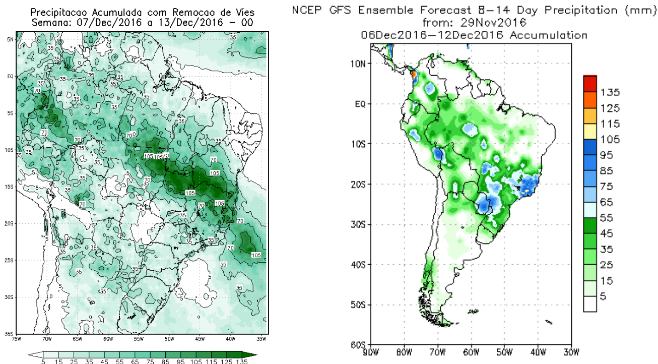
Figura 6. Previsão de precipitação em milímetros (mm) para a segunda semana, segundo a previsão por conjuntos do modelo numérico americano GFS/NCEP/NOAA (direita) e segundo o modelo brasileiro do CPTec-INPE-MCTI (esquerda).
