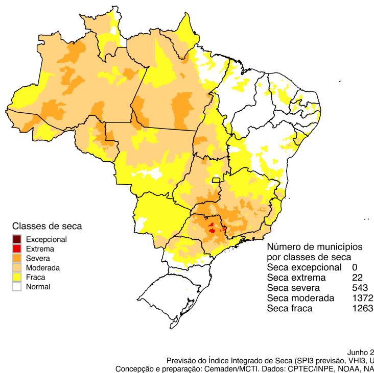
Figura 2 - Previsão do Índice Integrado de Seca (IIS3) para o mês de junho de 2024.
