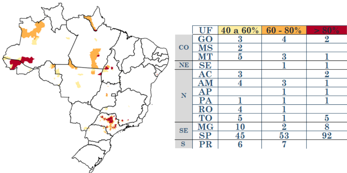
Figura 3 - Municípios com pelo menos 40% de área impactada pela seca (considerando apenas as áreas de pastagens e agrícolas) de acordo com o IIS-3, referente a situação em maio de 2024 para o Brasil.
