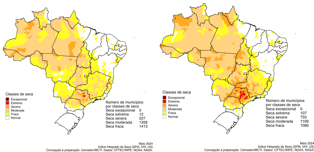
Figura 1 - Índice Integrado de Seca (IIS) referente ao mês de maio de 2024 nas escalas de 3 meses (IIS3, esquerda) e 6 meses (IIS6, direita).
