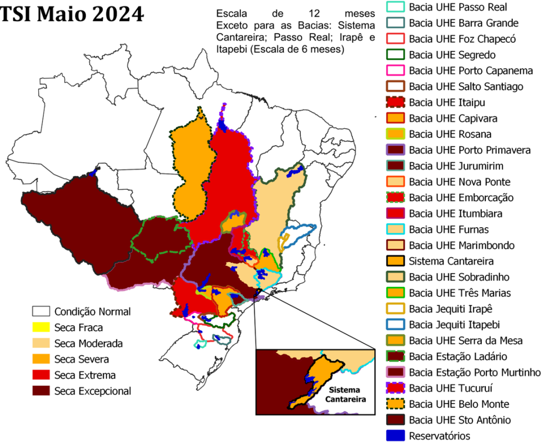
Figura 4 - Índice Padronizado Bivariado (Chuva-Vazão) - TSI-12 (Two-variate Standardized Index) - para o mês de maio. As delimitações coloridas representam as principais bacias monitoradas ao longo do país com suas respectivas classes de seca (variando de excepcional a seca fraca) e à condição dentro da normalidade. Fonte dos dados entre Jan/1981-Maio/2024: Precipitação (CHIRPS); e Vazão (Agência Nacional de Águas e Saneamento Básico -ANA/Operador Nacional do Sistema Elétrico -ONS).
