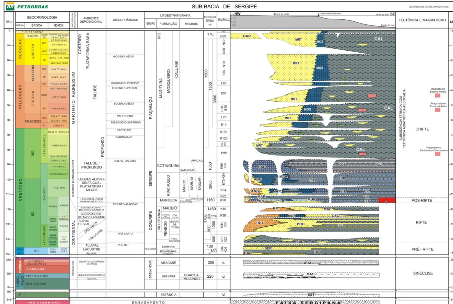
Figura 4. Diagrama estratigráfico da Sub-bacia de Sergipe (Campos Neto et al., 2007).
