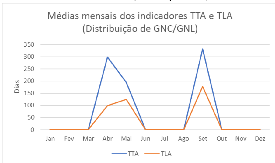
Gráfico 20 - Indicadores TTA e TLA para Instalações de GNC/GNL em 2023
