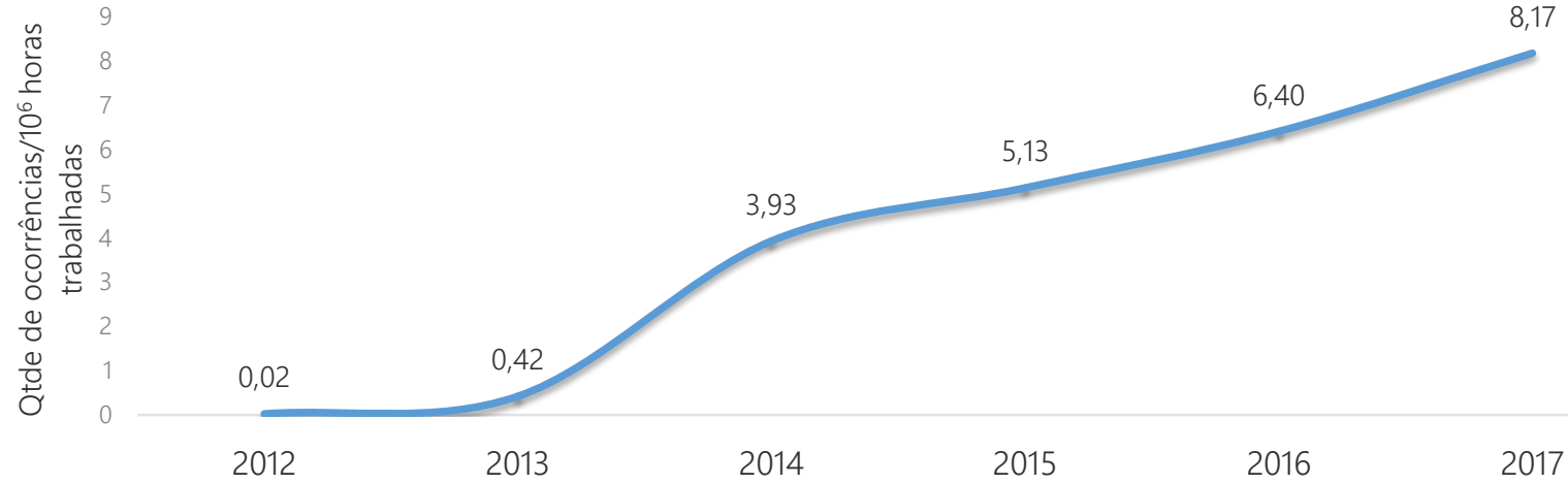
Falhas no BOP em sondas de perfuração marítimas
