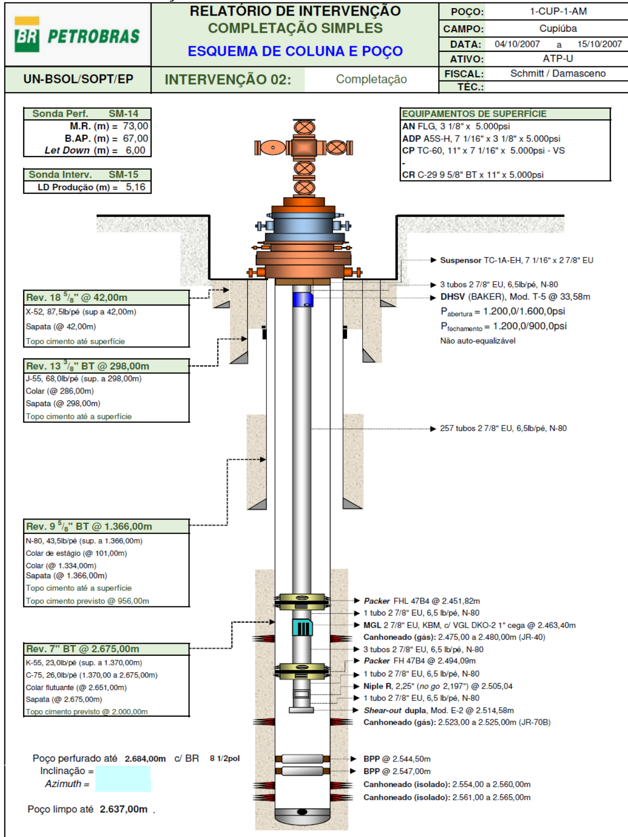
Imagem 3: Esquema mecânico do poço 1-CUP-01-AM
