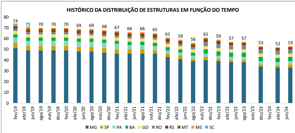
Figura 3 - Histórico da distribuição de estruturas a montante inseridas na PNSB em função do tempo (dados de 01/07/24).
