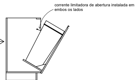
vista superior indicando sentido de abertura das portas
