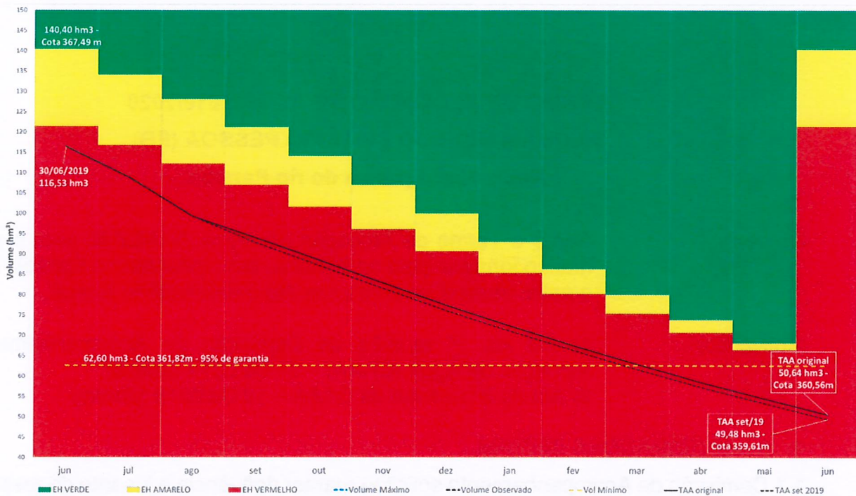
Figura 1 – cenários de volumes no reservatório Epitácio Pessoa (jun/19 a jun/20)
