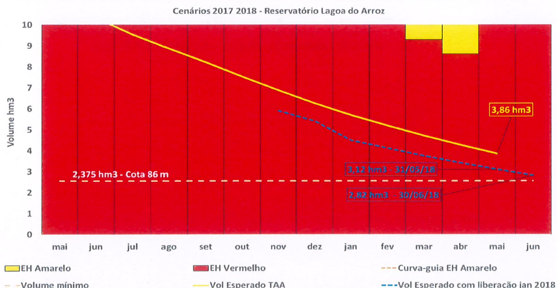
Figura 1 – Curvas de deplecionamento do açude Lagoa do Arroz indicando a situação esperada com o TAA original e com a liberação de água em janeiro de 2018
