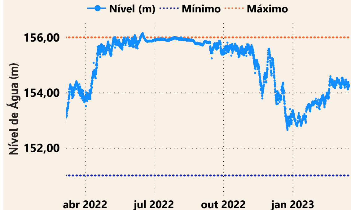
UHE Estreito Barramento (23490000)
