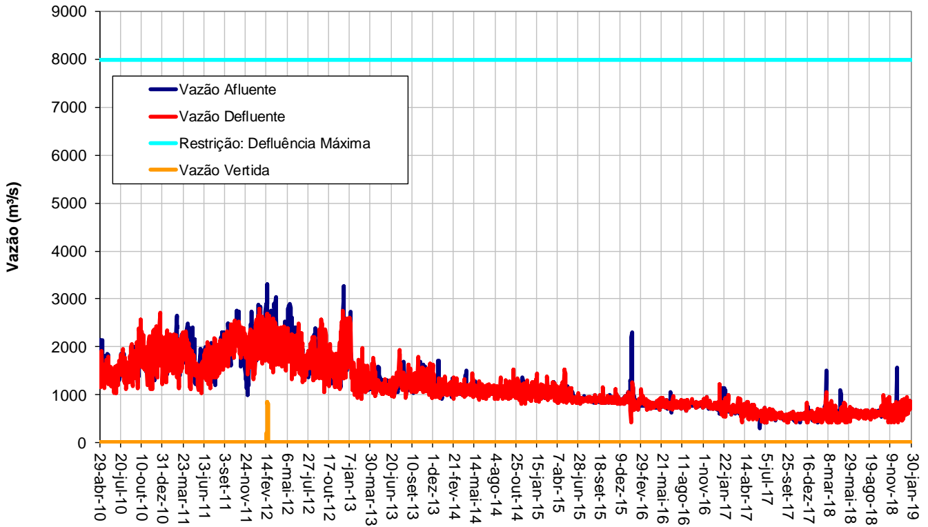
ITAPARICA - VAZÕES
