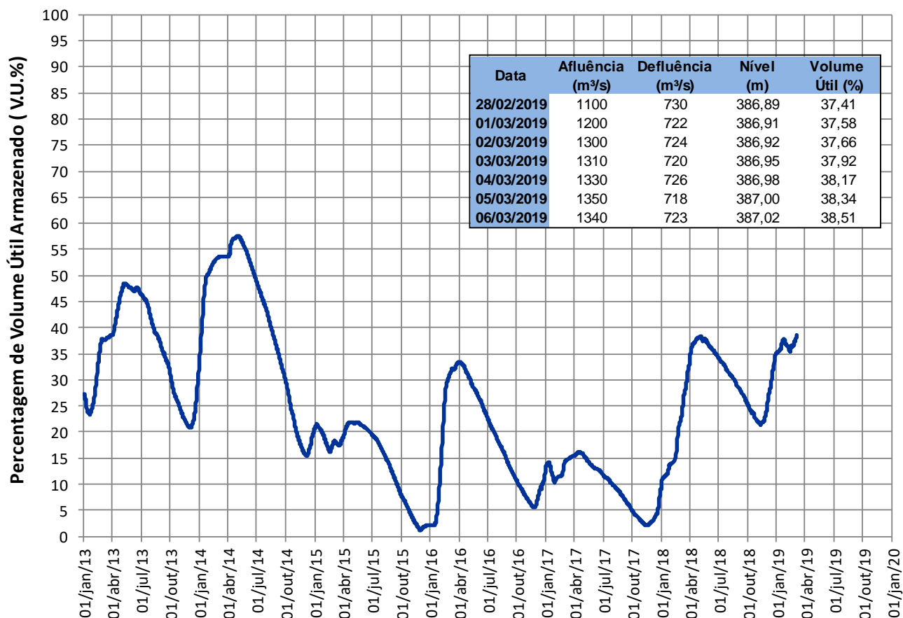
SOBRADINHO - VOLUME ÚTIL (%)
