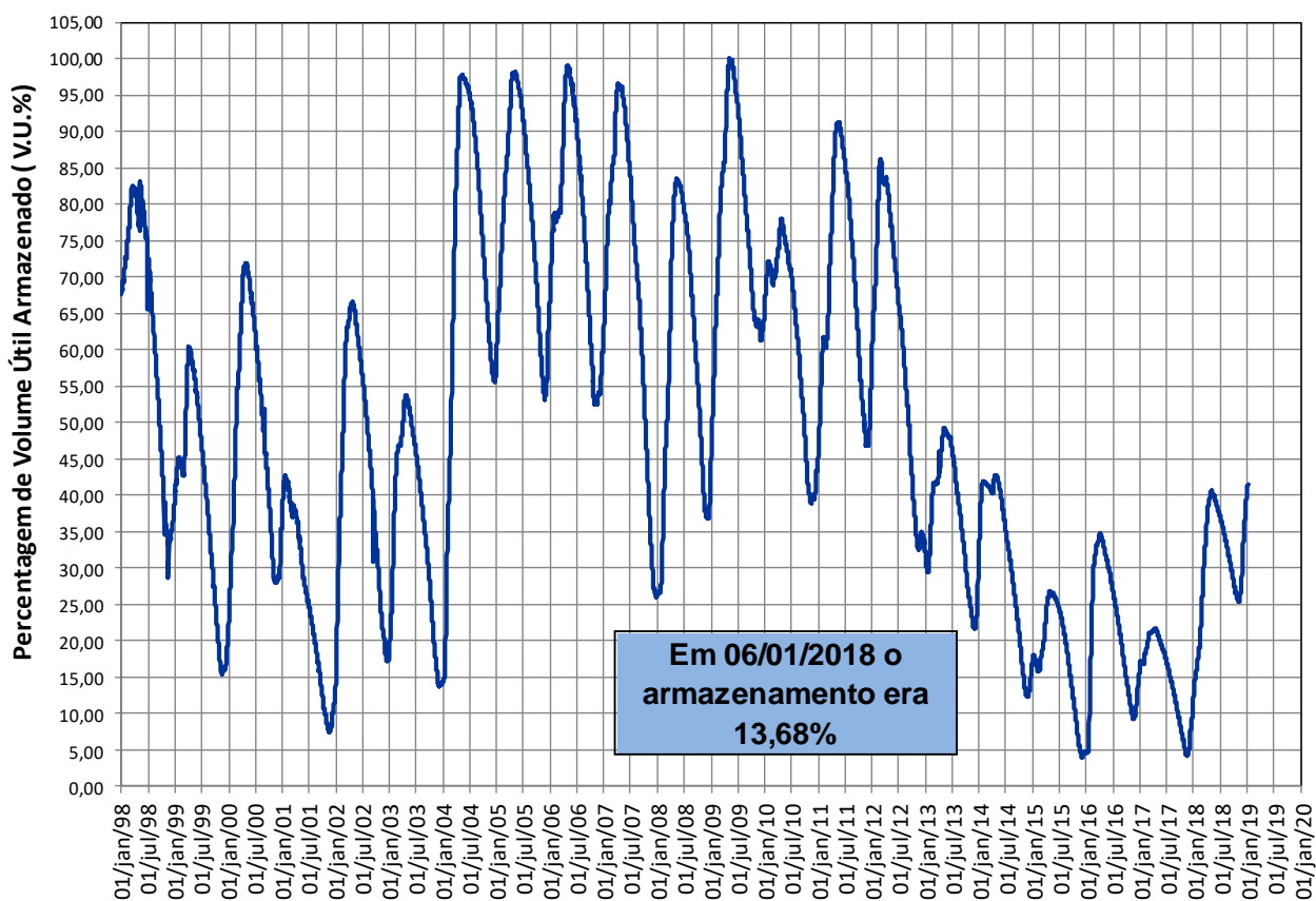
RESERVATÓRIO EQUIVALENTE - VOLUME ACUMULADO DESDE 1998
