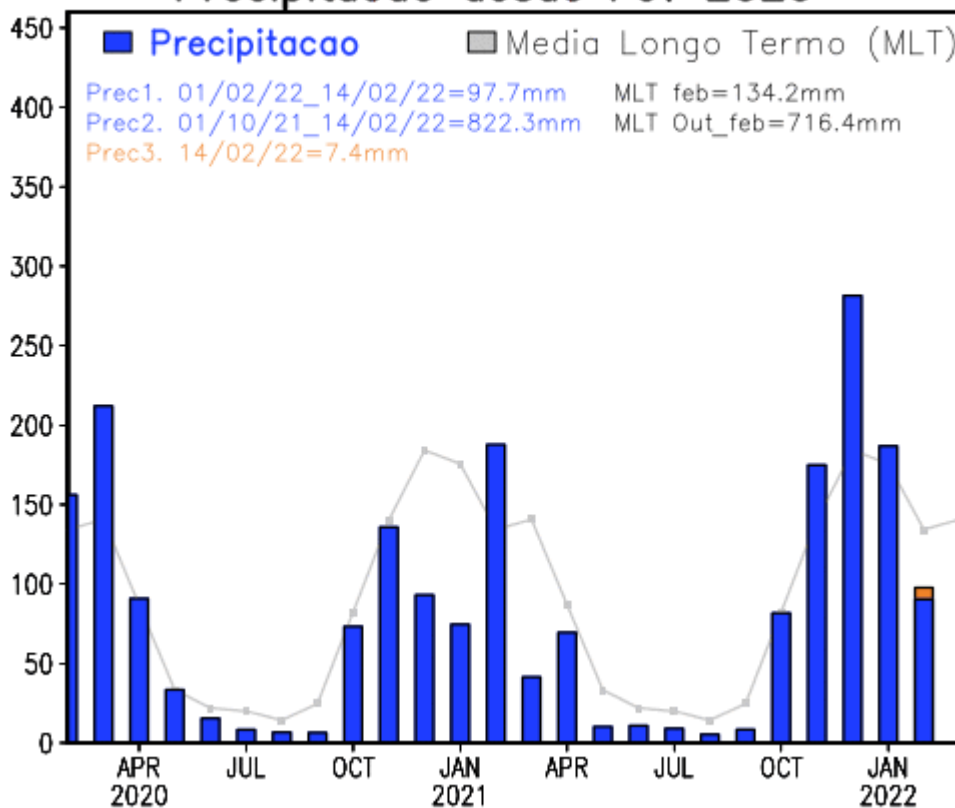
Precipitacao desde Feb 2020
