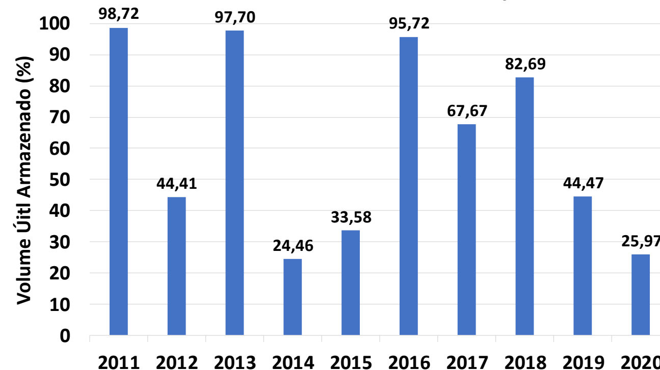
Volume Útil Armazenado em 18/05
