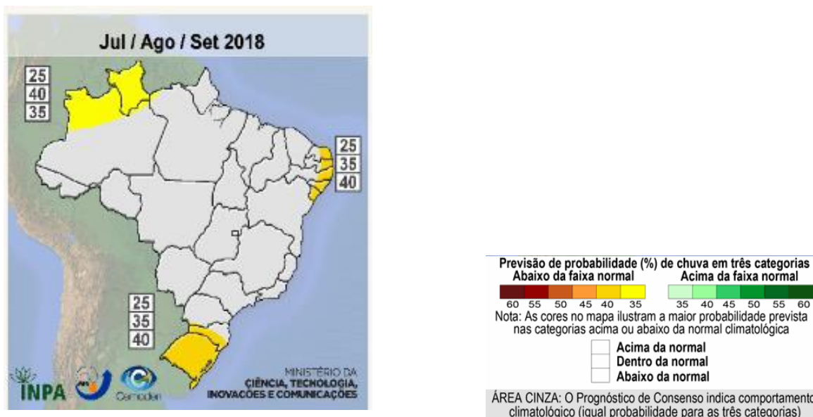
Figura 12 – Previsão climática para o trimestre Jul. a Set./2018.
