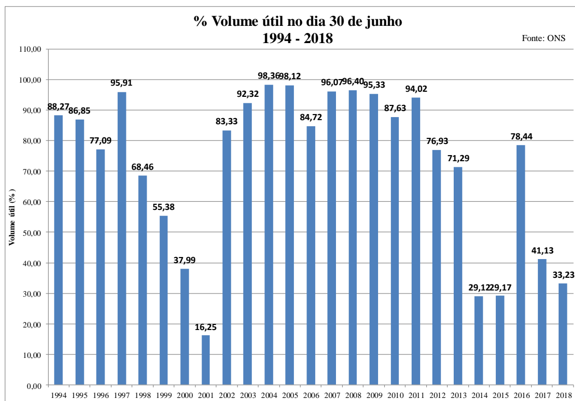
Figura 8 – Porcentagem do volume útil no dia 30 de junho, desde 1994 até 2018
