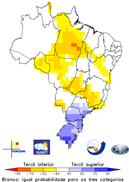
Figura 12 – Previsão climática sazonal por tercil (categorias abaixo, dentro e acima da faixa normal) para o trimestre set. a nov./2019.
