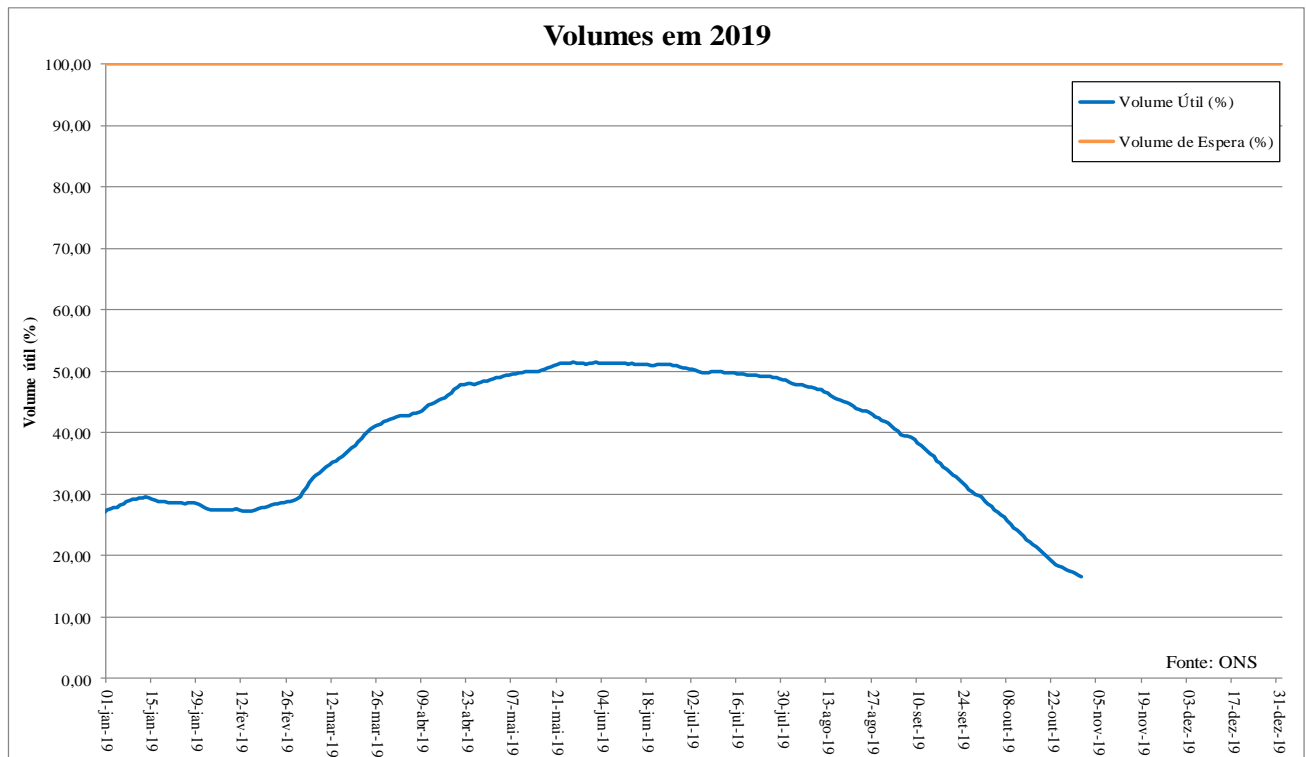
Figura 6 – Volumes no reservatório de Furnas em 2019
