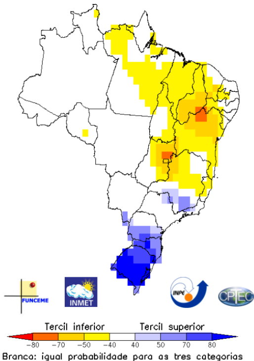
Figura 12 – Previsão climática sazonal por tercil (categorias abaixo, dentro e acima da faixa normal) para o trimestre nov./2019 a jan./2020.
