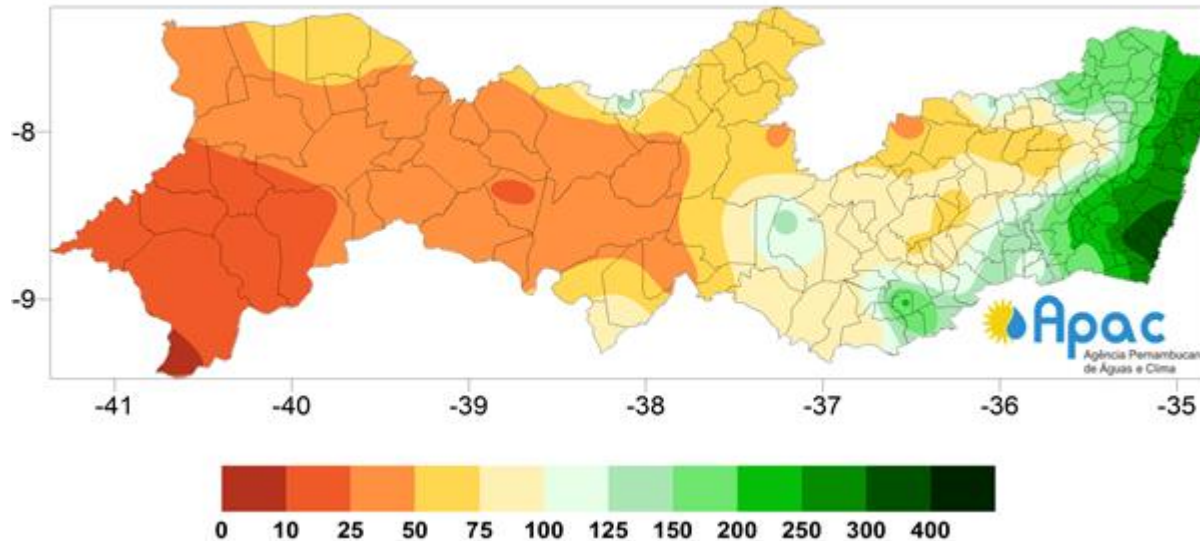
Climatologia da precipitação mensal (mm) Maio
