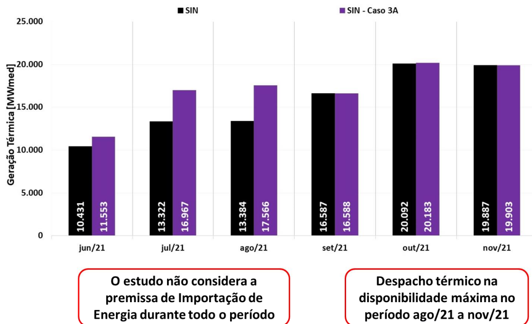
Figura 5-5: Geração Térmica do Cenário de Referência e do Cenário de Sensibilidade (Chuva 2020)
