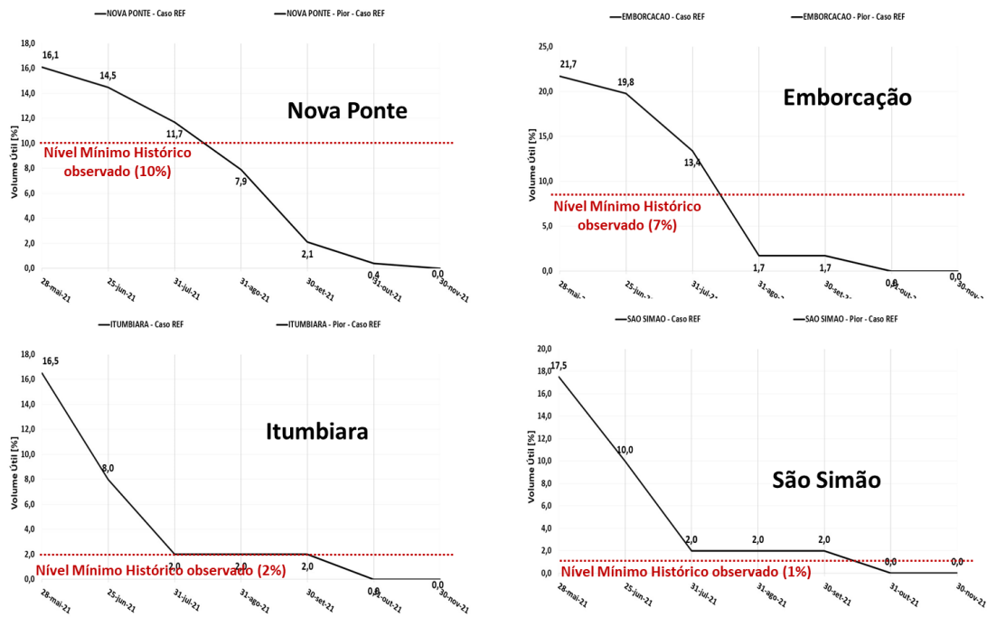
Figura 4-7: Volume Útil dos Principais Reservatórios da Bacia do Rio Paranaíba
