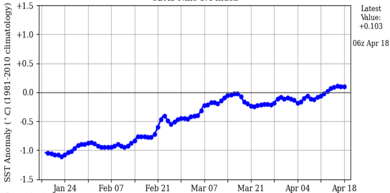
CDAS Niño 3.4 Index
