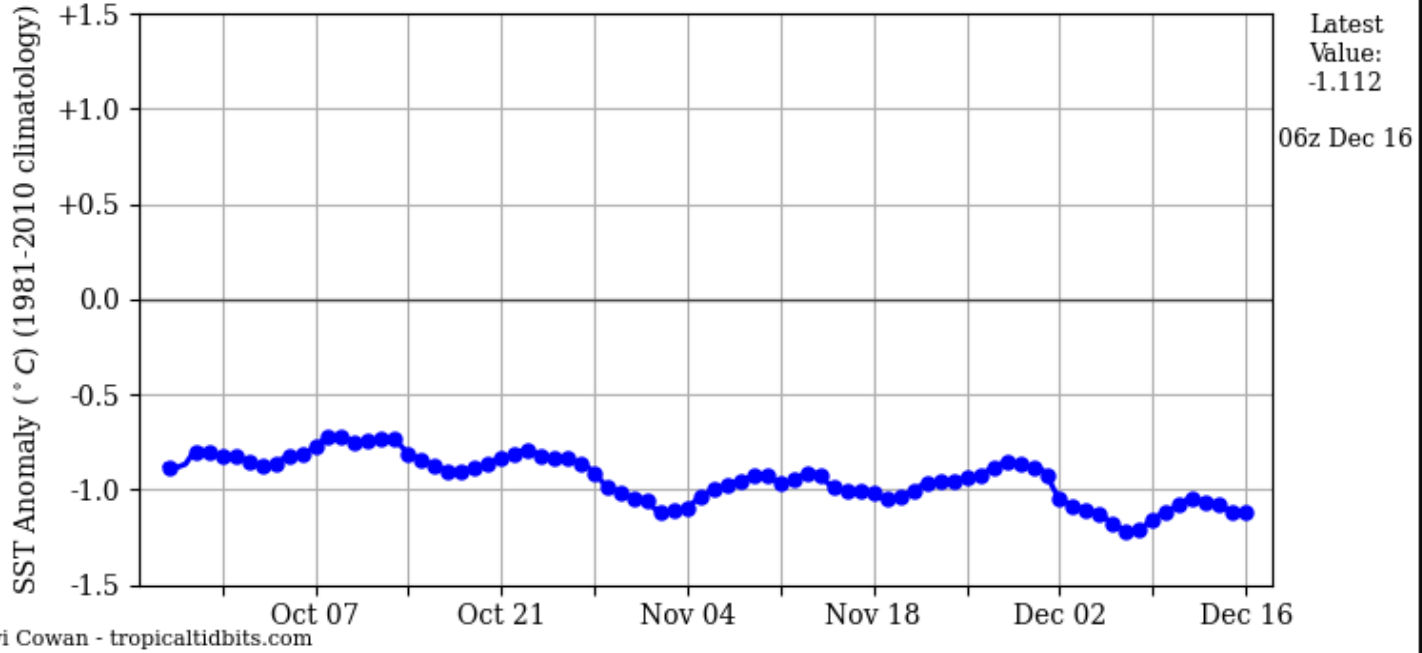
CDAS Niño 3.4 Index
