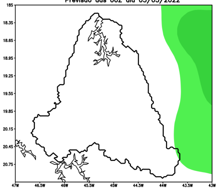
GEFS / Tres Marias Precipitacao acumulada em 7 dias (mm) Previsao das 00Z dia 03/05/2022
