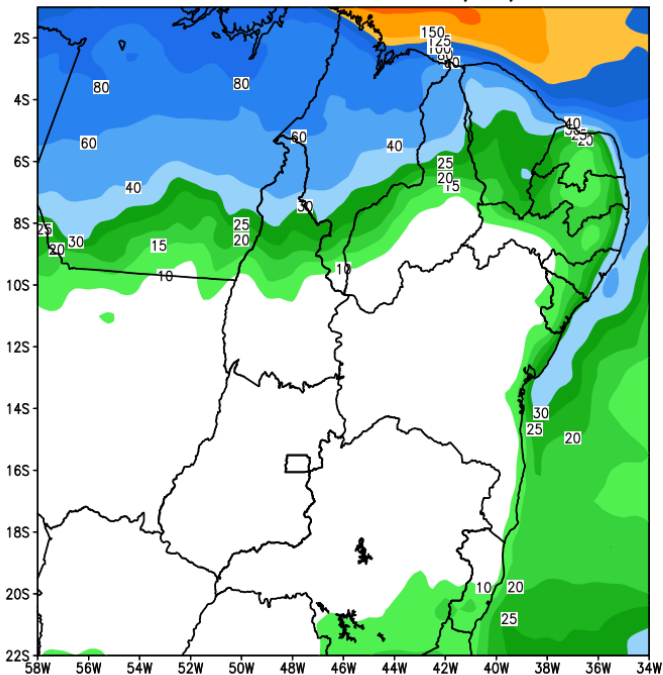
GEFS / BRASIL_NE Precipitacao acumulada 2aSem (mm) Previsao das 00Z dia 03/05/2022
