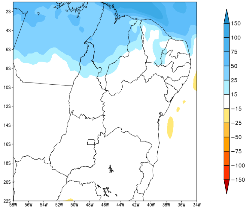
Anomalia de Precipitacao BR NE (mm) Periodo: 2022051100 a 2022051700
