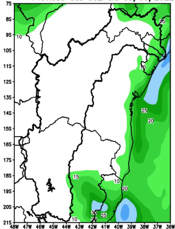
GEFS / Bacia do Rio Sao Francisco Precipitacao acumulada em 7 dias (mm) Previsao das 00Z dia 03/05/2022
