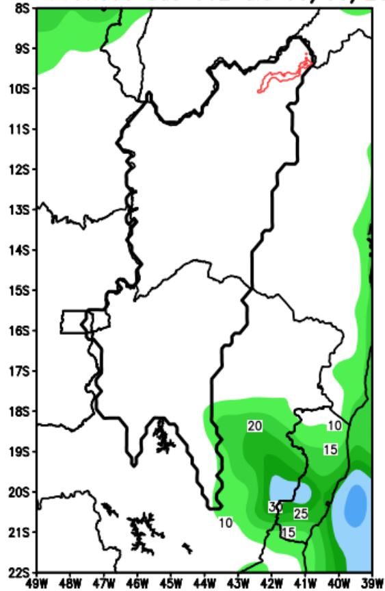
GEFS / Sobradinho Precipitacao acumulada em 7 dias (mm) Previsao das 00Z dia 03/05/2022
