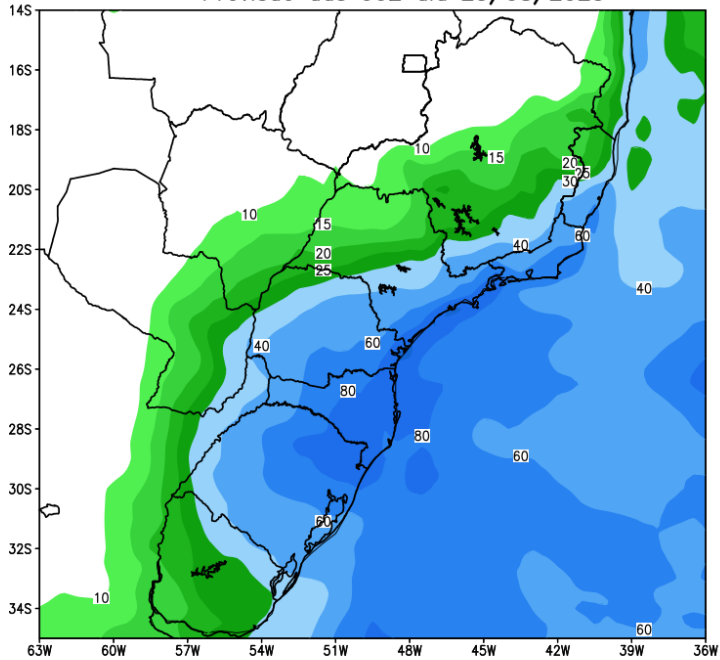
GEFS / BRASIL_SUL Precipitacao acumulada 14dias (mm) Previsao das 00Z dia 23/08/2023
