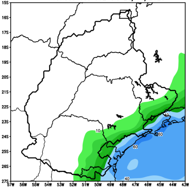
GEFS / Bacia do Parana Precipitacao acumulada em 7 dias (mm) Previsao das 00Z dia 23/08/2023
