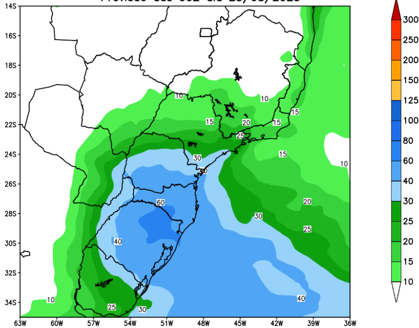
GEFS / BRASIL_SUL Precipitacao acumulada 2aSem (mm) Previsao das 00Z dia 23/08/2023
