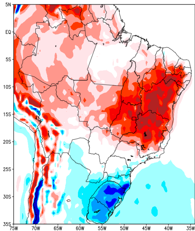
Anomalia de Temperatura BR (C) Período: 2023082300 a 2023083000
