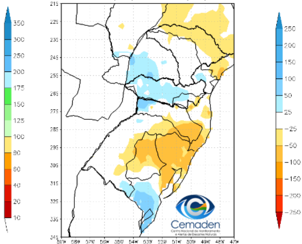
Anomalia de Precipitação (mm) A.S. Período: 23/07/2023 a 22/08/2023
