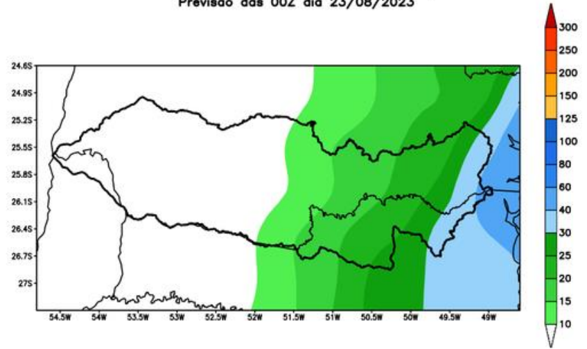
GEFS / Bacia do Rio Iguacu Precipitação acumulada em 7 dias (mm) Previsão das 00Z dia 23/08/2023
