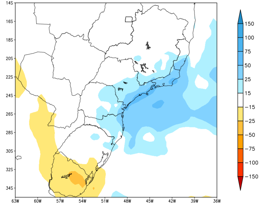
Anomalia de Precipitacao BR SUL (mm) Periodo: 2023082300 a 2023090600
