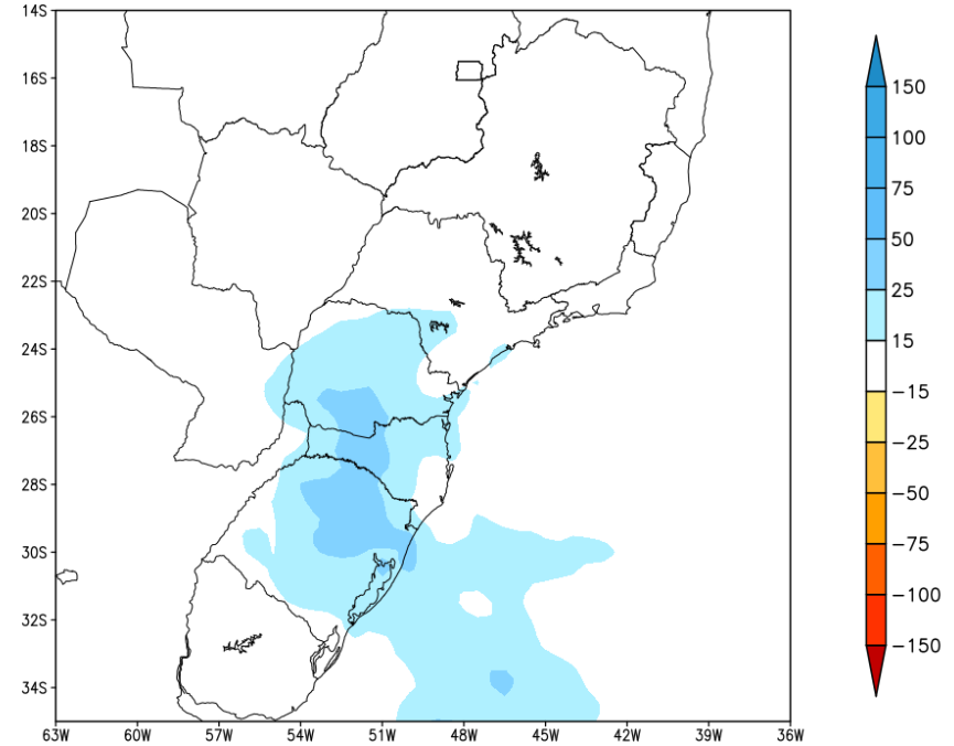
Anomalia de Precipitacao BR_SUL (mm) Periodo: 2023083100 a 2023090600
