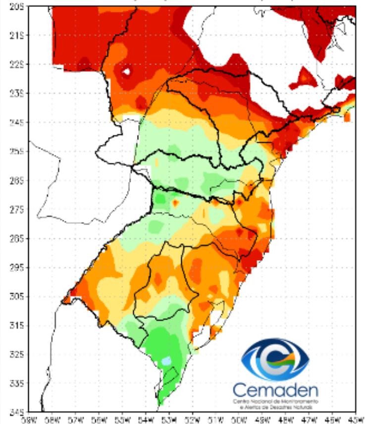
Precipitação Acumulada (mm) A.S. Período: 23/07/2023 a 22/08/2023
