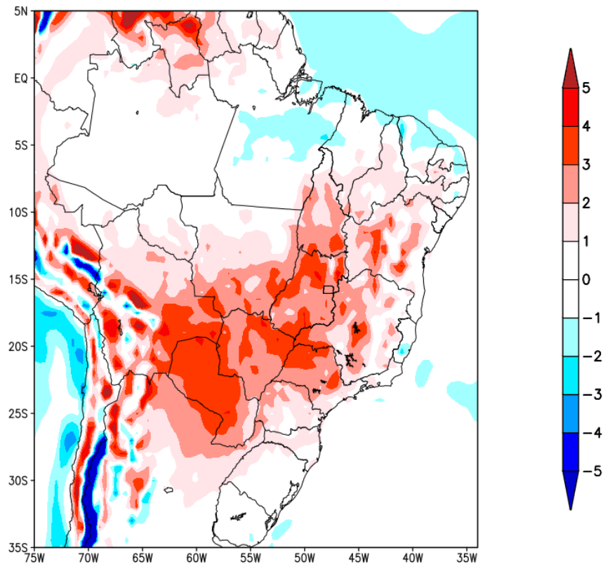
Anomalia de Temperatura BR (C) Período: 2023083100 a 2023090600
