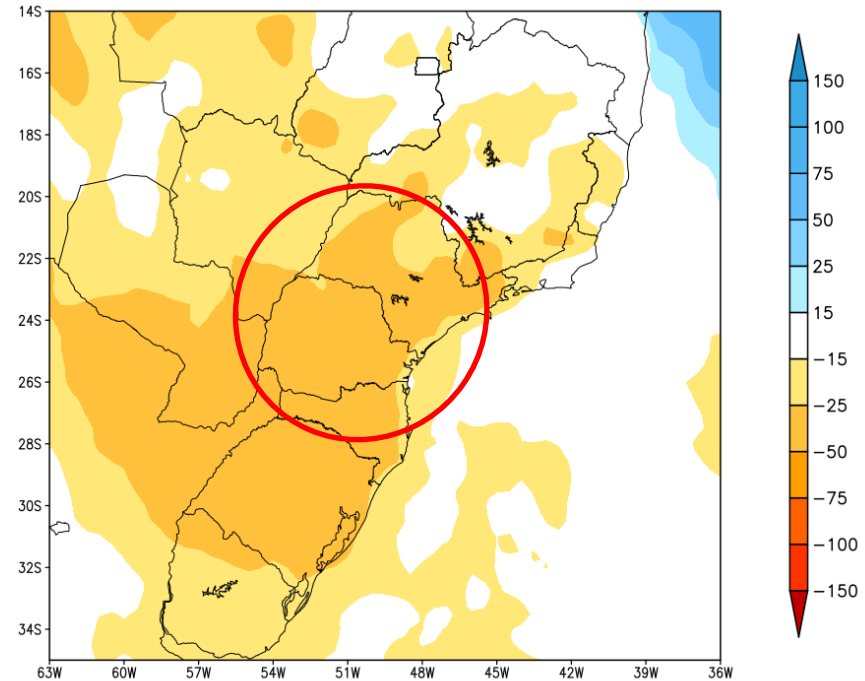
Anomalia de Precipitacao BR_SUL (mm) Periodo: 2022110400 a 2022111000
