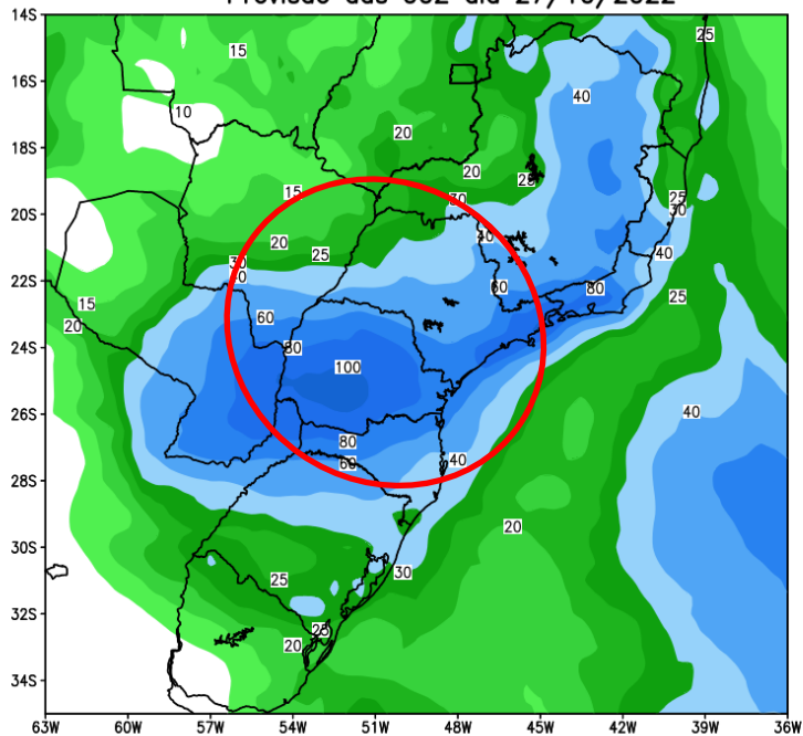
GEFS / BRASIL_SUL Precipitacao acumulada 1aSem (mm) Previsao das 00Z dia 27/10/2022
