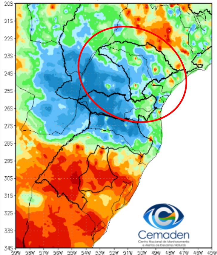
Precipitação Acumulada (mm) A.S. Período: 26/09/2022 a 26/10/2022
