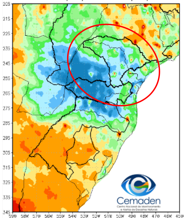
Precipitação Acumulada (mm) A.S. Período: 27/08/2022 a 26/10/2022
