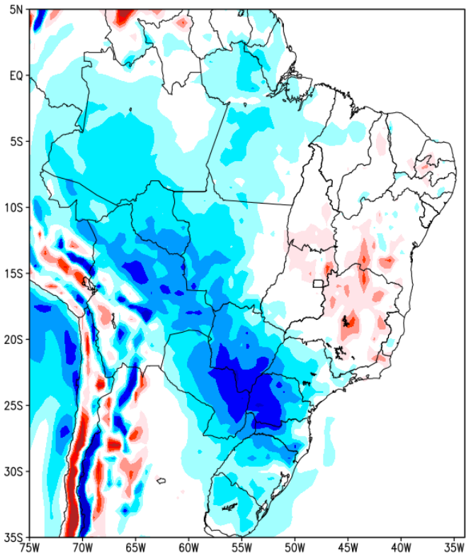
Anomalia de Temperatura BR (C) Período: 2022102700 a 2022110300
