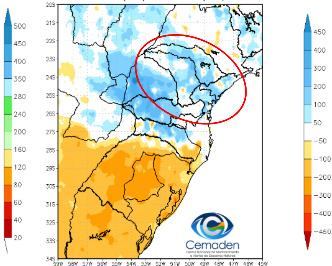
Anomalia de Precipitação (mm) A.S. Período: 27/08/2022 a 26/10/2022
