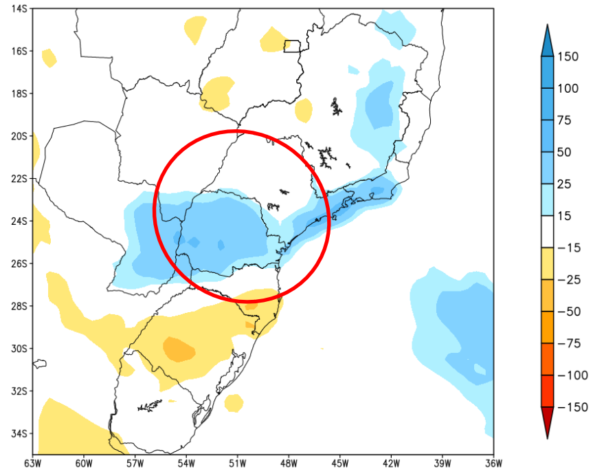
Anomalia de Precipitacao BR_SUL (mm) Periodo: 2022102700 a 2022110300
