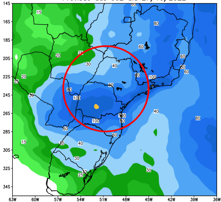
GEFS / BRASIL_SUL Precipitacao acumulada 14dias (mm) Previsao das 00Z dia 27/10/2022
