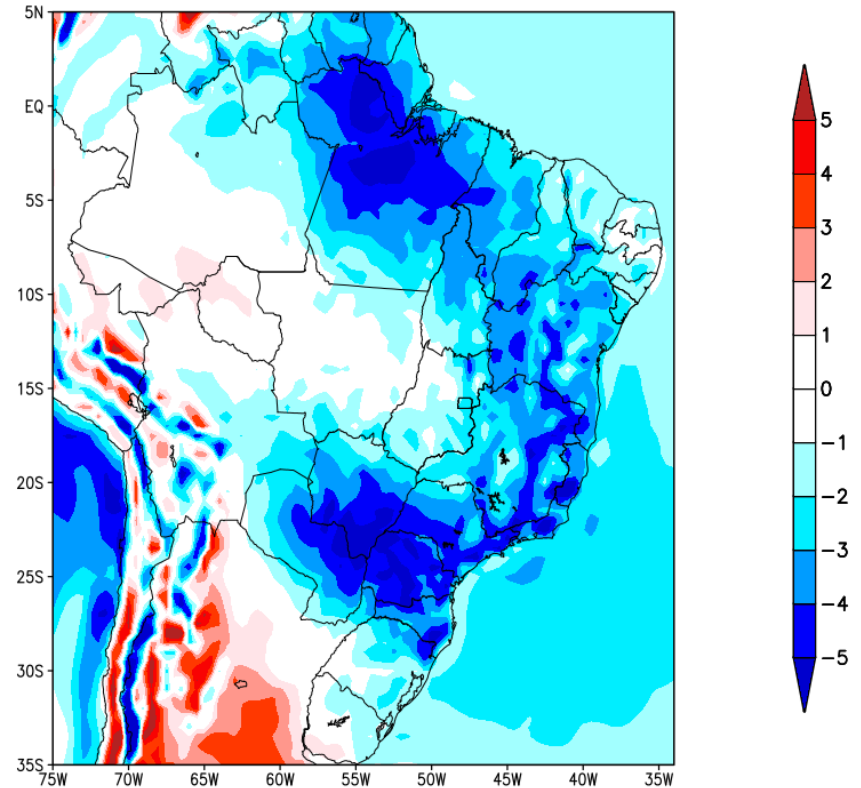
Anomalia de Temperatura BR (C) Período: 2022110400 a 2022111000
