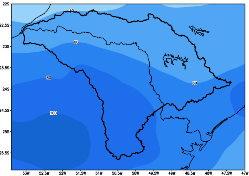
GEFS / Bacia do Rio Paranapanema Precipitacao acumulada em 7 dias (mm) Previsao das 00Z dia 27/10/2022
