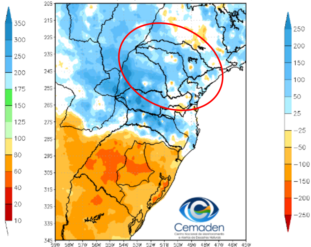
Anomalia de Precipitação (mm) A.S. Período: 26/09/2022 a 26/10/2022
