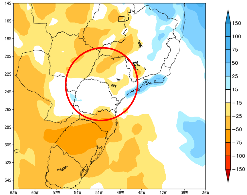
Anomalia de Precipitacao BR_SUL (mm) Periodo: 2022102700 a 2022111000
