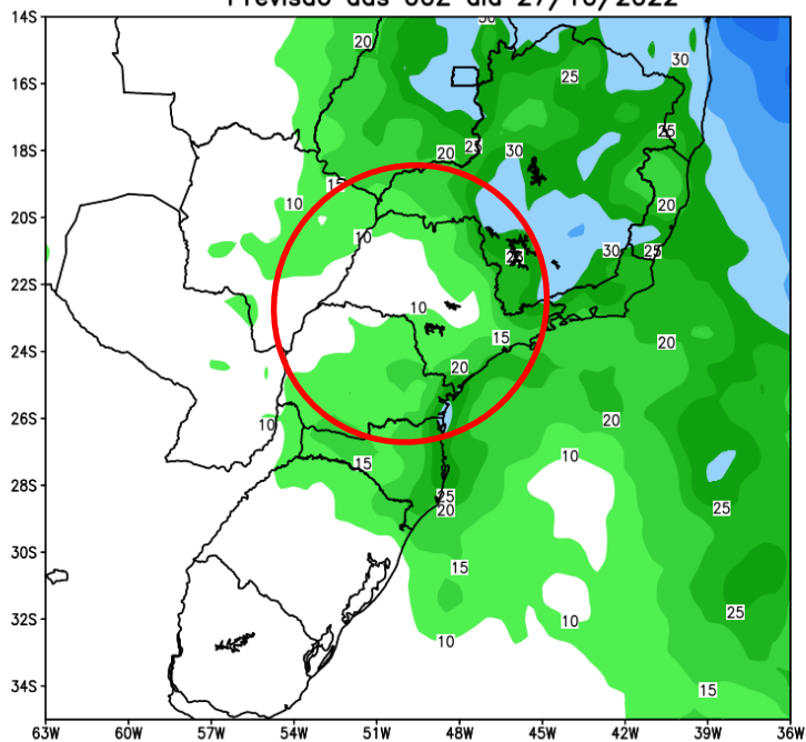
GEFS / BRASIL_SUL Precipitacao acumulada 2aSem (mm) Previsao das 00Z dia 27/10/2022
