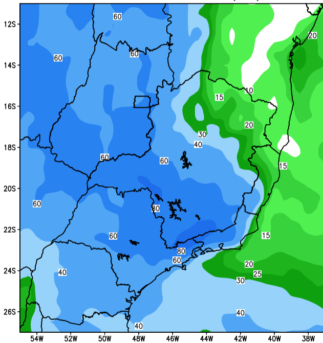
GEFS / BRASIL_SE Precipitacao acumulada 2aSem (mm) Previsao das 00Z dia 14/02/2023
