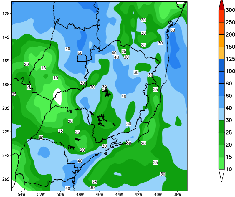
GEFS / BRASIL_SE Precipitacao acumulada 1aSem (mm) Previsao das 00Z dia 12/04/2022
