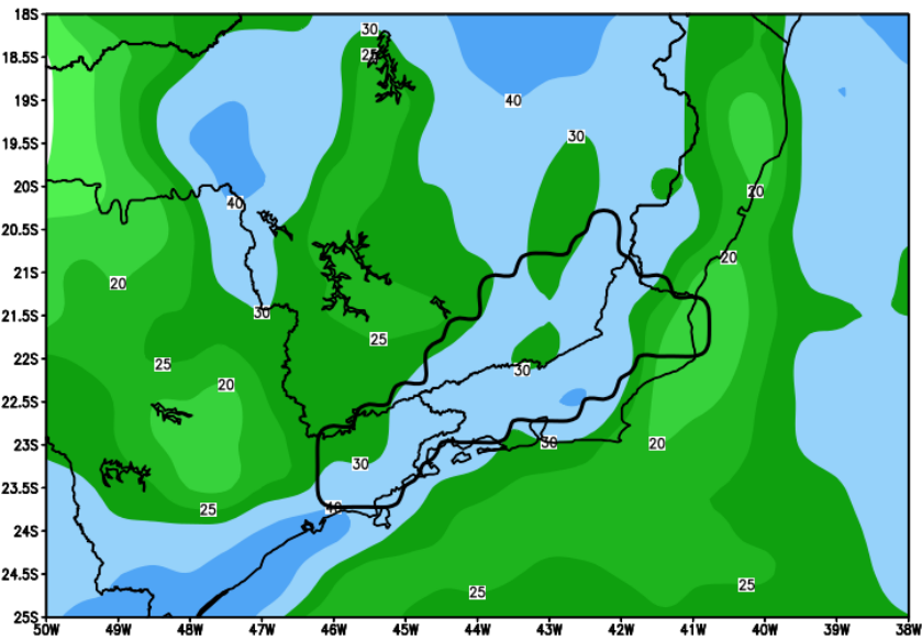
GEFS / Bacia do Rio Paraíba do Sul Precipitacao acumulada em 7 dias (mm) Previsao das 00Z dia 12/04/2022
