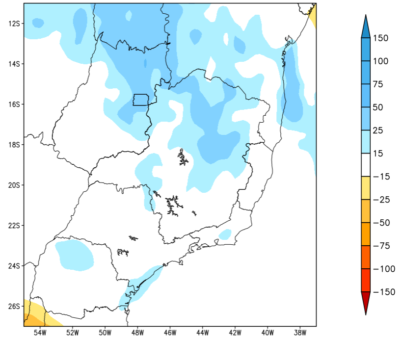
Anomalia de Precipitacao BR SE (mm) Periodo: 2022041200 a 2022041900
