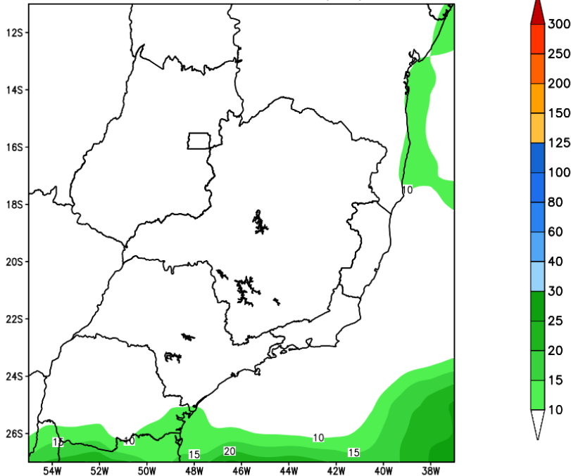
GEFS / BRASIL_SE Precipitacao acumulada 1aSem (mm) Previsao das 00Z dia 11/07/2023
