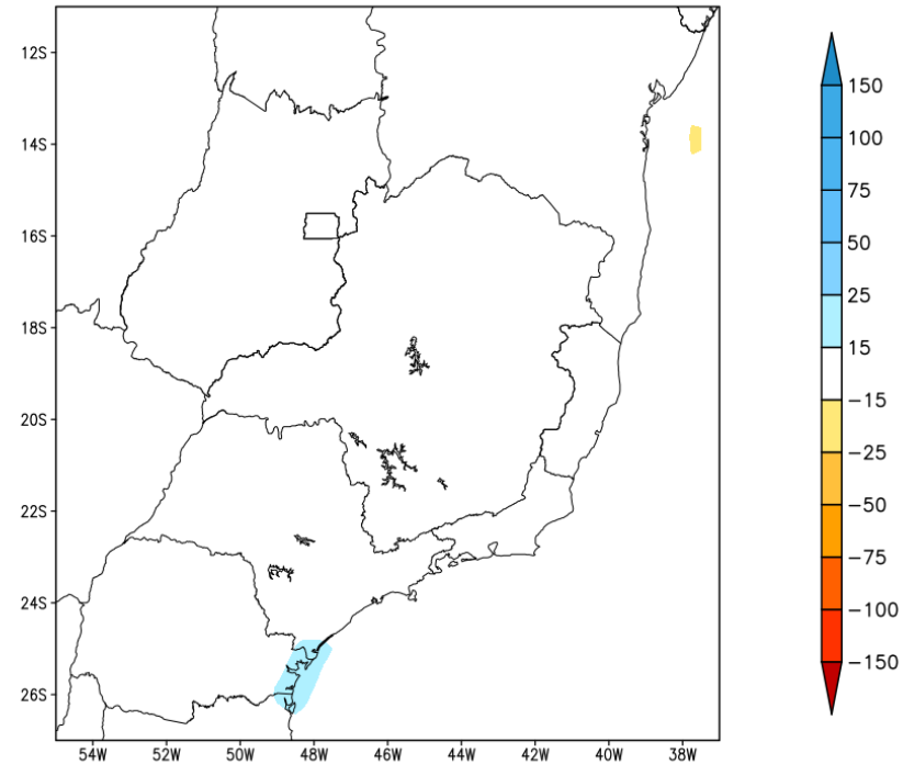
Anomalia de Precipitacao BR_SE (mm) Periodo: 2023071900 a 2023072500
