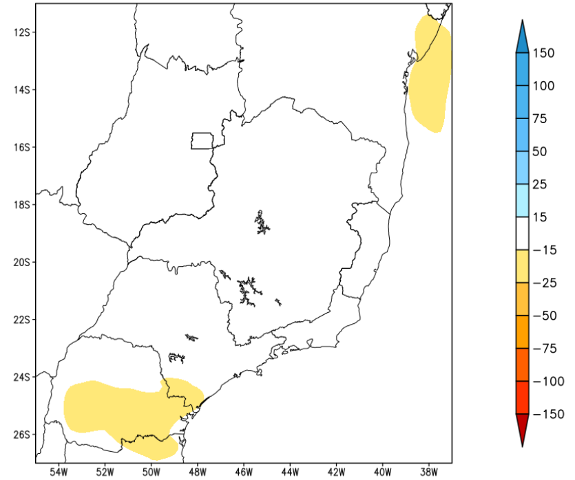
Anomalia de Precipitacao BR_SE (mm) Periodo: 2023071100 a 2023071800
