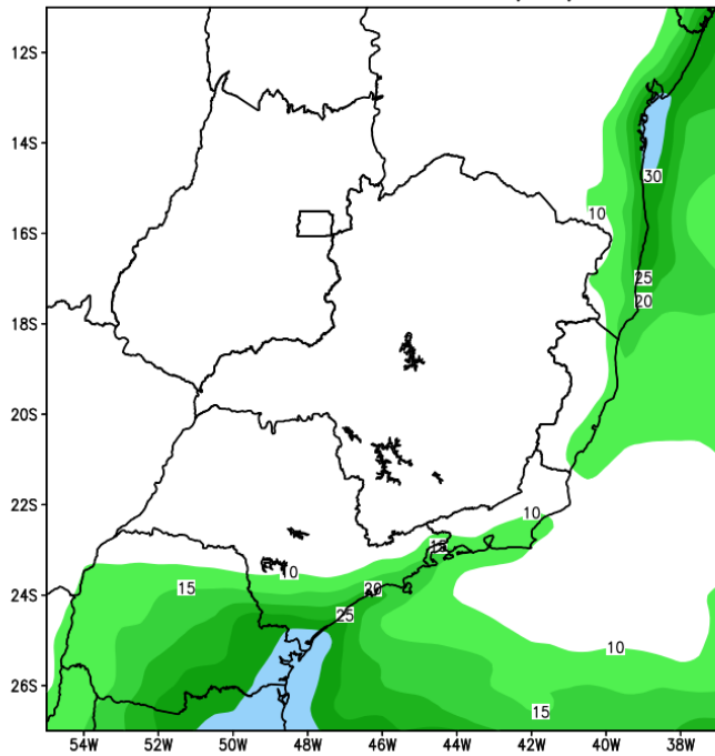
GEFS / BRASIL_SE Precipitacao acumulada 2aSem (mm) Previsao das 00Z dia 11/07/2023
