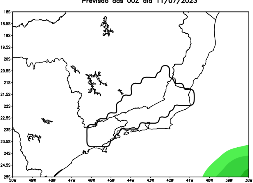
GEFS / Bacia do Rio Paraíba do Sul Precipitacao acumulada em 7 dias (mm) Previsao das 00Z dia 11/07/2023
