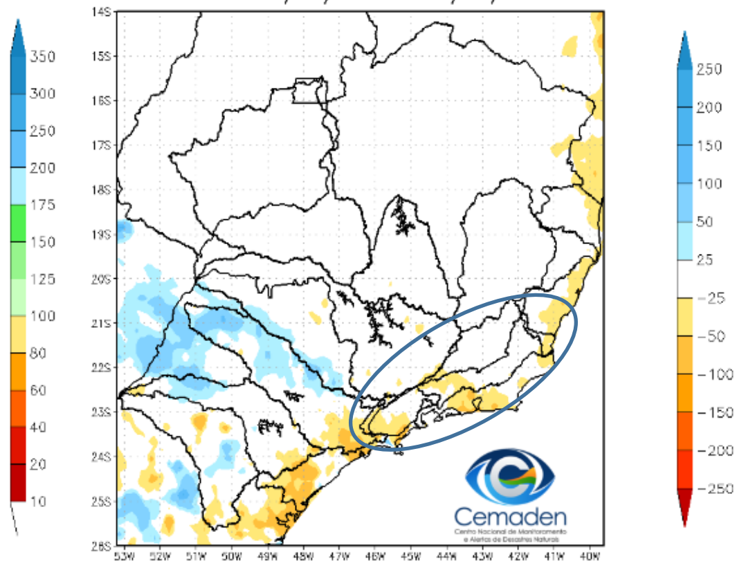
Anomalia de Precipitação (mm) A.S. Período: 10/06/2023 a 10/07/2023
