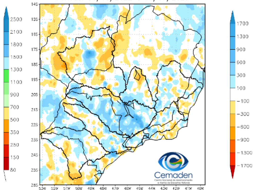
Anomalia de Precipitação (mm) A.S. Período: 01/10/2022 a 10/07/2023
