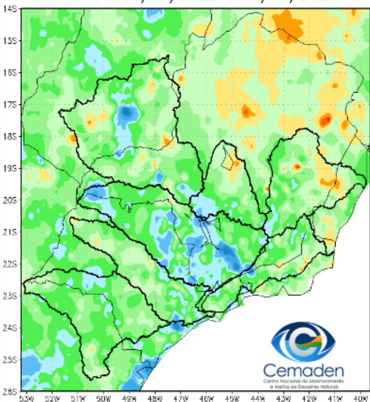
Precipitação Acumulada (mm) A.S. Período: 01/10/2022 a 10/07/2023
