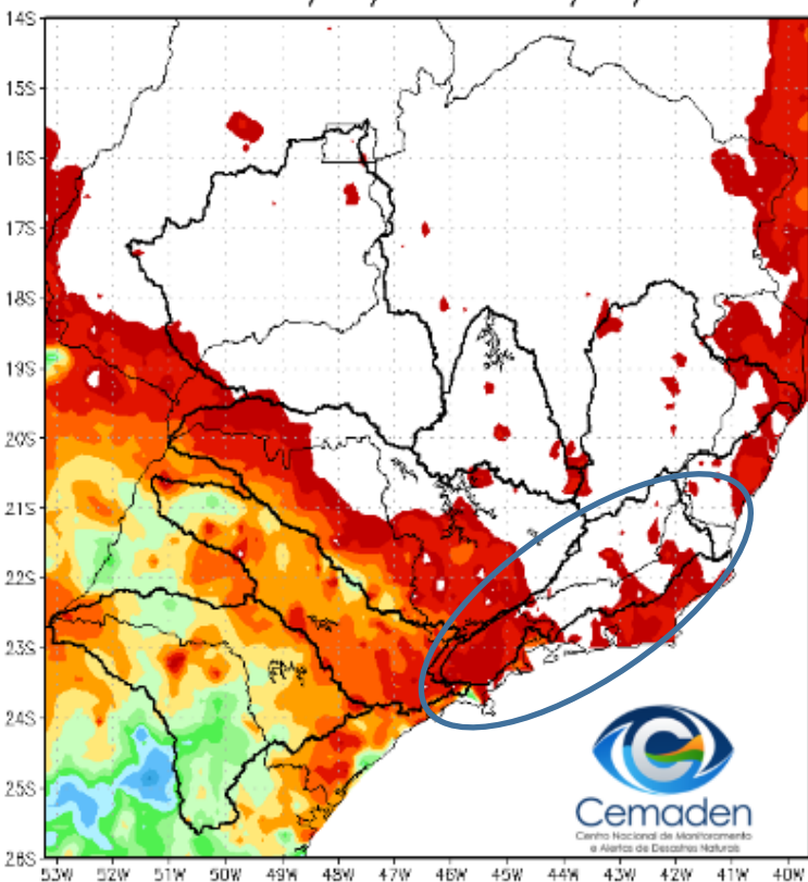
Precipitação Acumulada (mm) A.S. Período: 10/06/2023 a 10/07/2023
