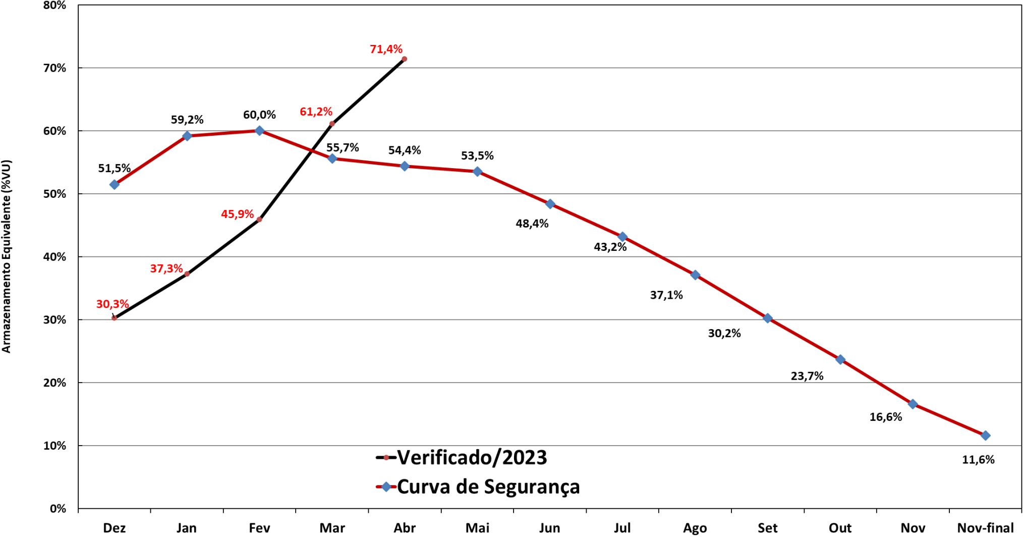
Curva de Segurança para Operação Normal - Paraíba do Sul
